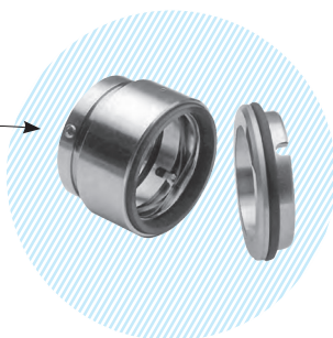
Jednoduchá o-kroužková ucpávka, INDUSERV 24, typ VJ920N
